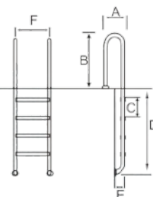
Събми за бассейн, модел Narrow - с фланци за монтаж
