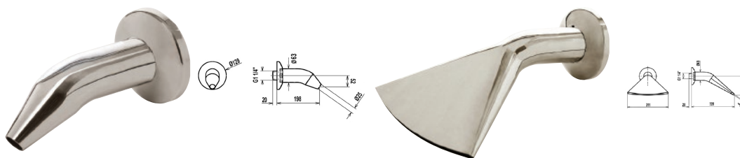
Дюзи за масаж, Flexinox. Изработени от неръждаема стомана AISI316.
