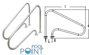
Перило за басейн с анкери за вграждане
