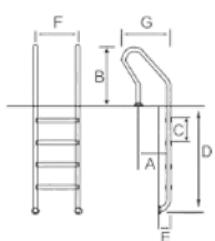
Събми за бассейн, модел Squint - с фланци за монтаж
