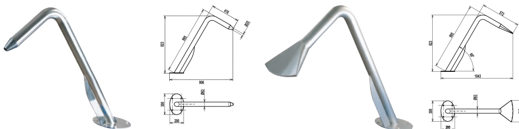
Водно оръдие, модел Fiji, Flexinox. Изработено от неръждаема стомана AISI316.
